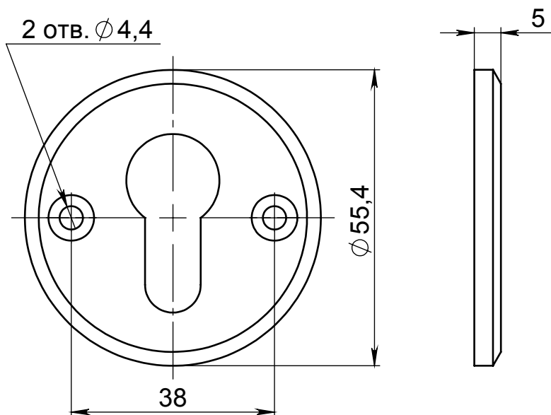
Накладка декоративная
